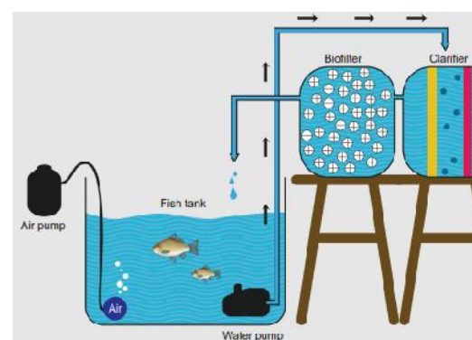
Figura 1.4 - Sistema di Acquacoltura a ricircolo
