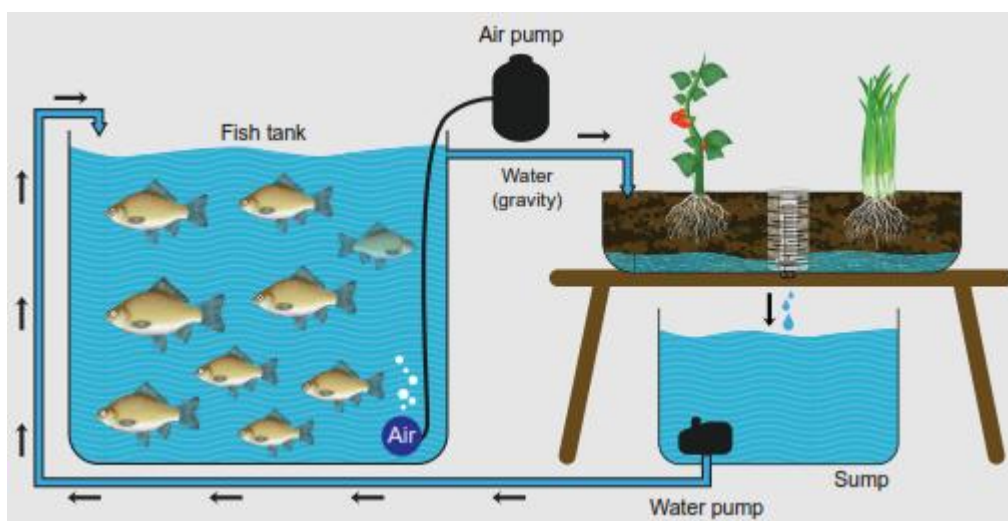
Figura 1.5 - Schema semplificato di una unità acquaponica
